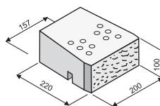
Geogarden stone štípaný
