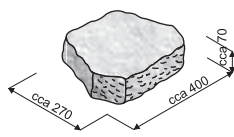
Nášlapný kámen malý
