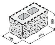
KB 13-21 B 400 RUSTIK
