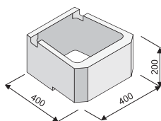
CUP STONE VELKÝ – provedení hladké
