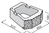
GEOSTONE® - SHELF štípaný
