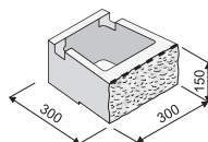
CUP STONE MALÝ – provedení štípané rustik
