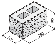
KB 13-21 B 350 GRIND
