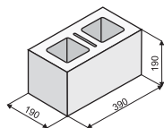
KB 1-20 A dělitelná
