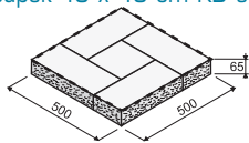
KB sh-50 G tl. 65 mm
