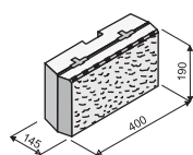
Pohledový prvek 400 štípaný
