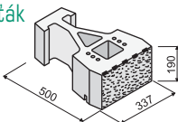
GEOSTONE® - FLAT tříčtvrták štípaný
