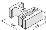
GEOSTONE® - FLAT hladký
