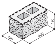
KB 13-21 B 400 GRIND
