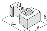
GEOSTONE® - FLAT tříčtvrták hladký
