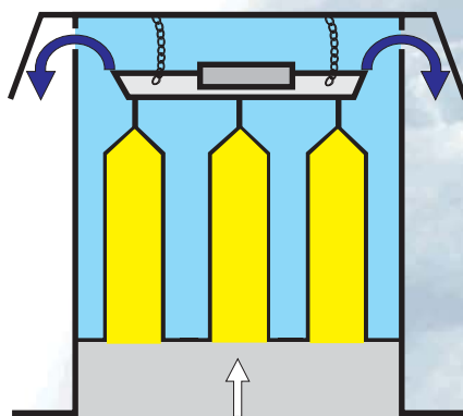
příčný řez filtrem
